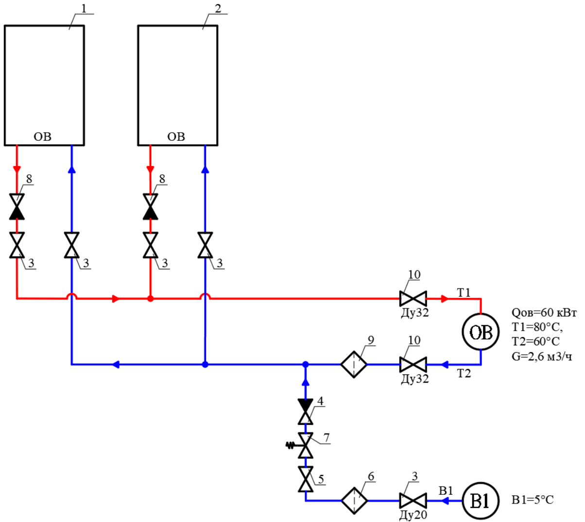
Тепломеханическая схема
