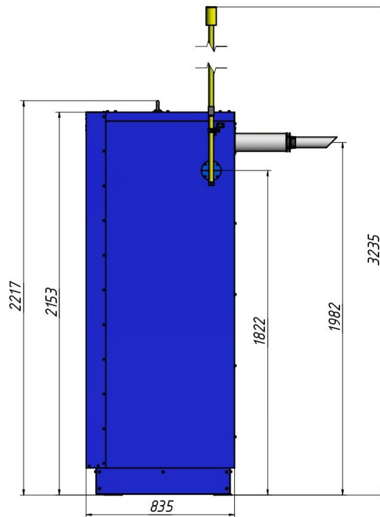
Вид слева без опции РДГ
