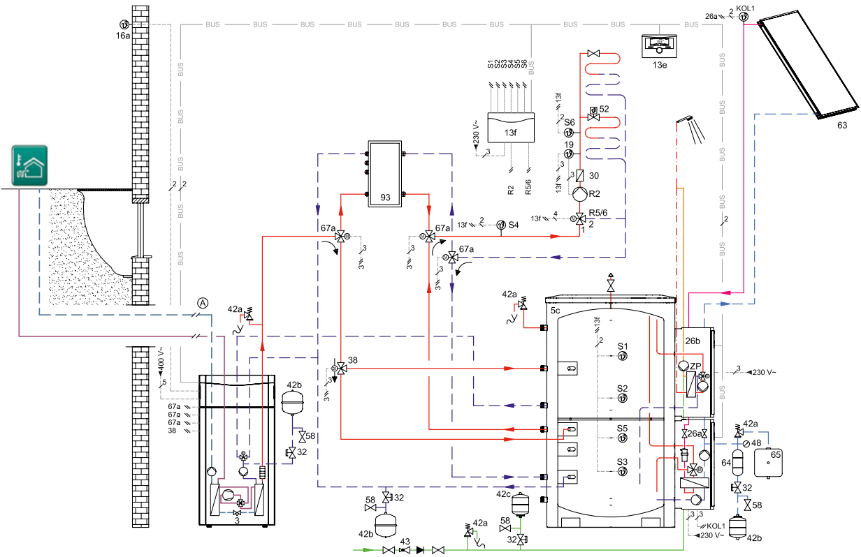
Схема 5 – Отопление с использованием солнечных панелей (auroTHERM)
