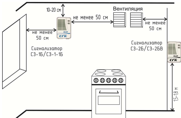
Рисунок.6. - Схема размещения сигнализаторов загазованности СЗ-Б.
