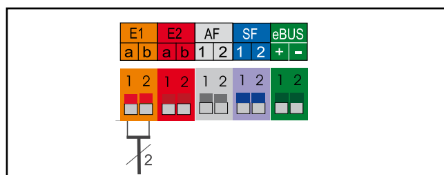
Подсоединение входа E1
