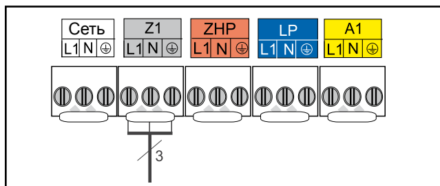
Подсоединение выхода Z1
