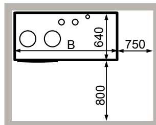
Котел в котельном помещении
