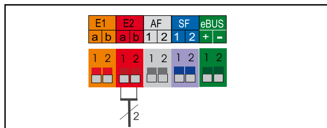
Подсоединение входа E2
