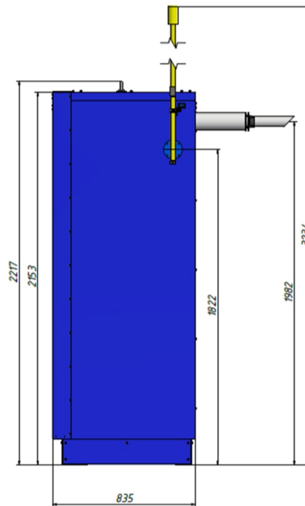
Вид справа
