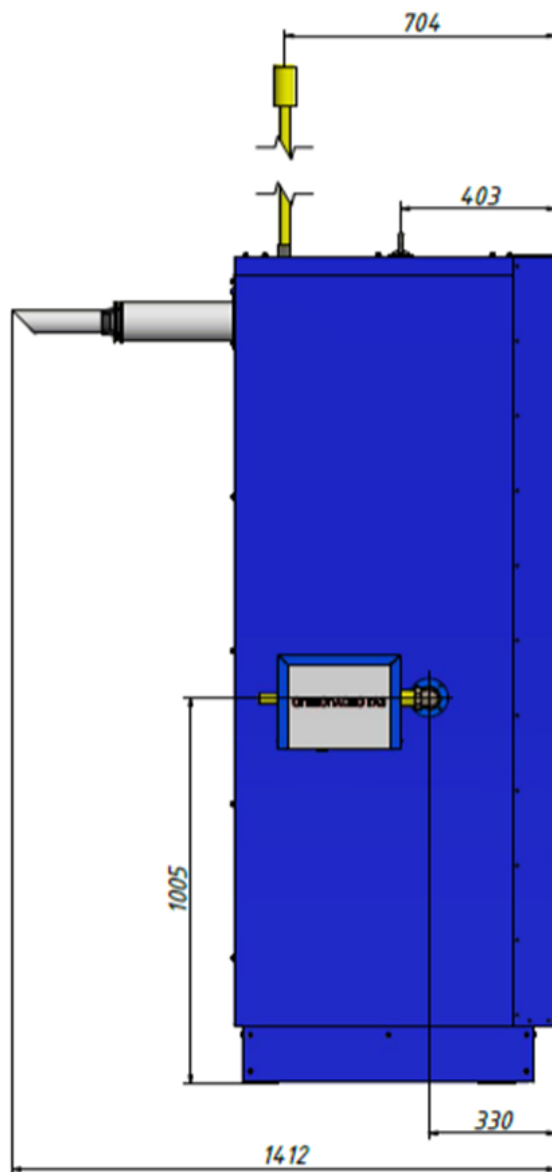
Вид слева с опцией РДГ
