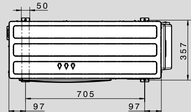
Наружный блок BWL-1S(B)-07 Вид сверху
