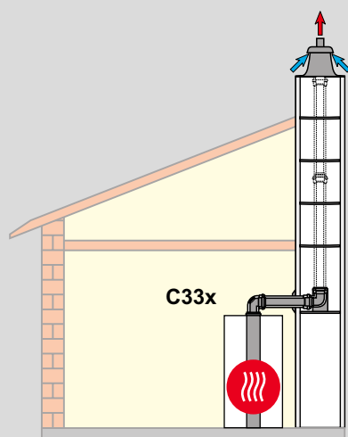
Комплект с концентрическим подключением DN60/100 к концентрической дымоходной трубе в шахте для режима подачи воздуха для горения из атмосферы
