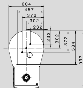
CSZ-2R Вид сверху
