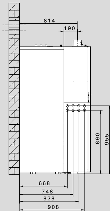
CSZ-2R Вид сбоку
