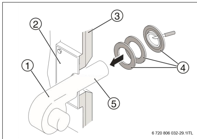
Рисунок 19 Монтаж горелки
