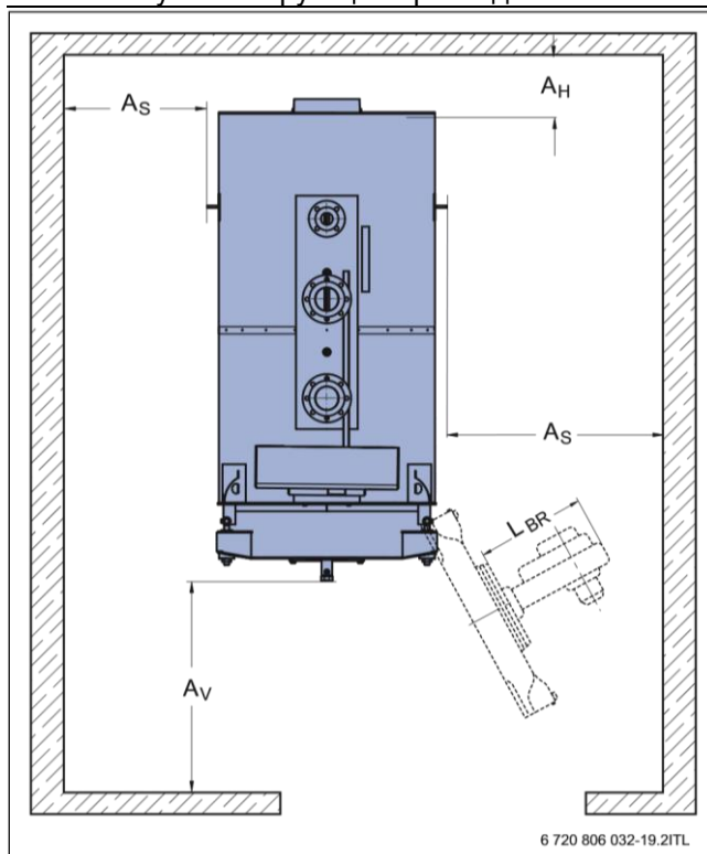
Рисунок 11 Помещение для установки котла (размеры в мм)
