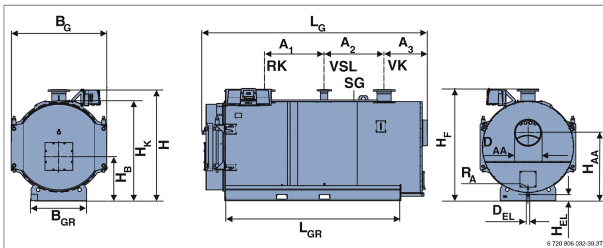
Рисунок 4 Размеры котлов SK 1400 – 2000 кВт
