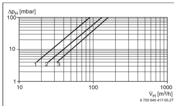
Рисунок 7 Гидравлическое сопротивление котлов SK 730 - 2000 кВт
